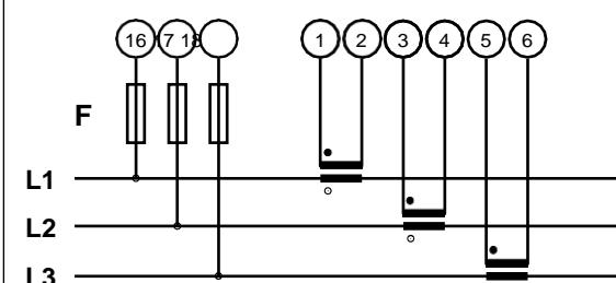
Trifase, 3 fili, connessione con 3 TA
