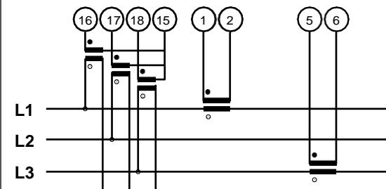
Trifase, 3 fili, connessione con 2 TA e 3 TV (Aron)
