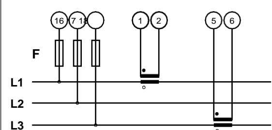
Trifase, 3 fili, connessione con 2 TA (Aron)
