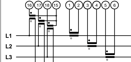
Trifase, 3 fili, connessione con 3 TA e 3 TV
